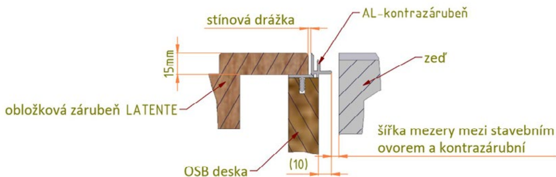
Detail horizontálního řezu
