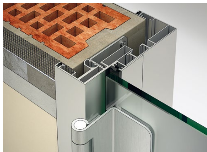
DYNAMIK pro stěny tl. 85–210 mm
