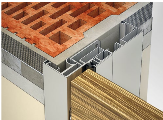
DYNAMIK pro stěny tl. nad 210 mm
